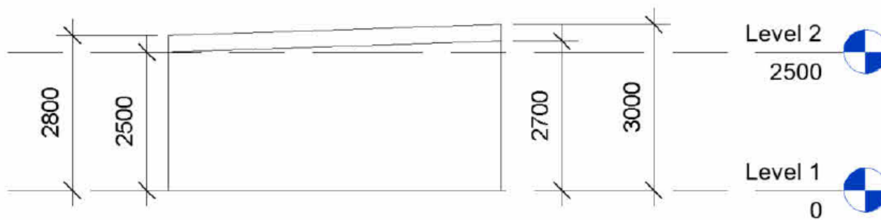
Facade syd
